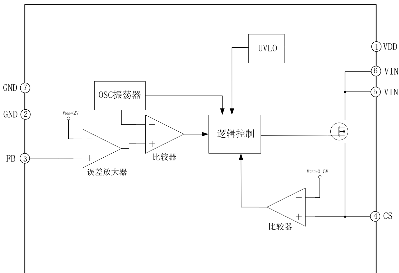
图 5-1. EG1177 内部电路图
