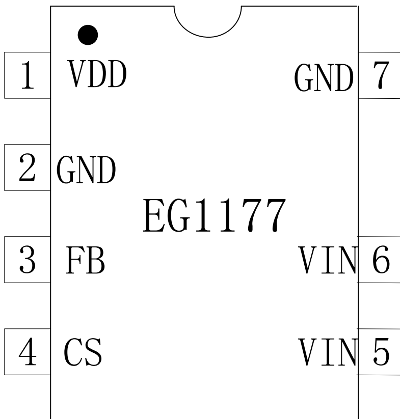
图 4-1. EG1177 管脚定义
