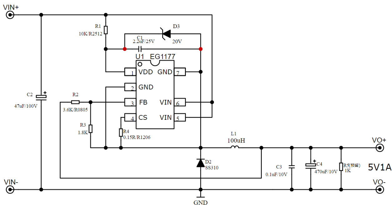
图 6-2. EG1177 5V 输出应用图
