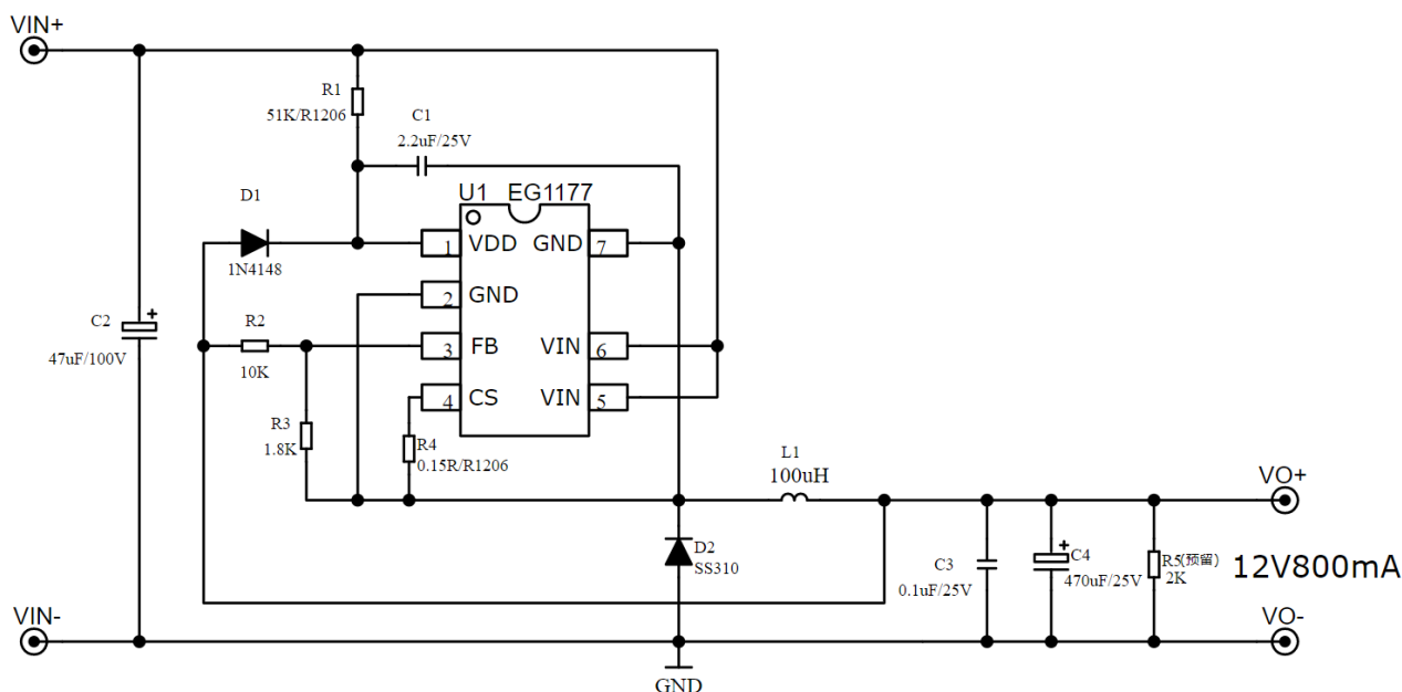
图 6-1. EG1177 12V 输出应用图
