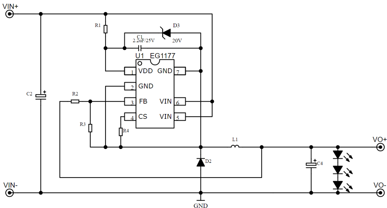
图 6-3. EG1177 LED 驱动应用图
